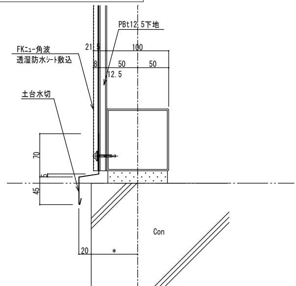
土台水切詳細図
