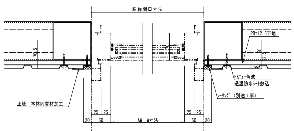
サッシ廻り(横断面)詳細図
