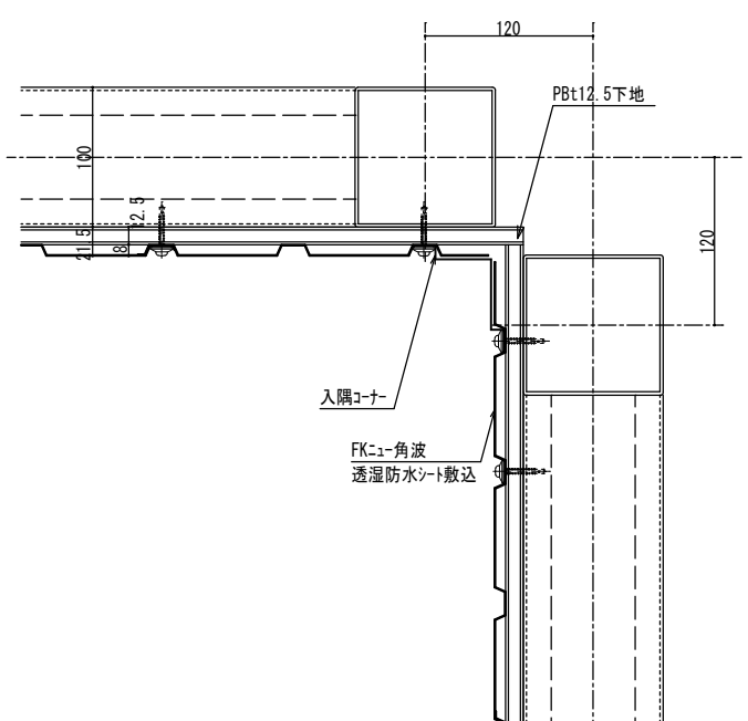
入隅コーナー詳細図
