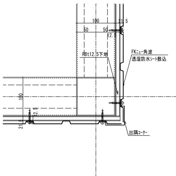
出隅コーナー詳細図
