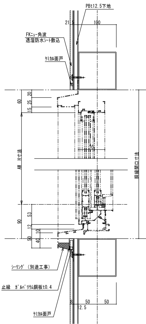
サッシ廻り(縦断面)詳細図
