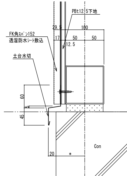
土台水切詳細図
