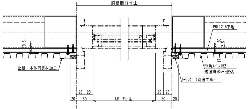
サッシ廻り(横断面)詳細図
