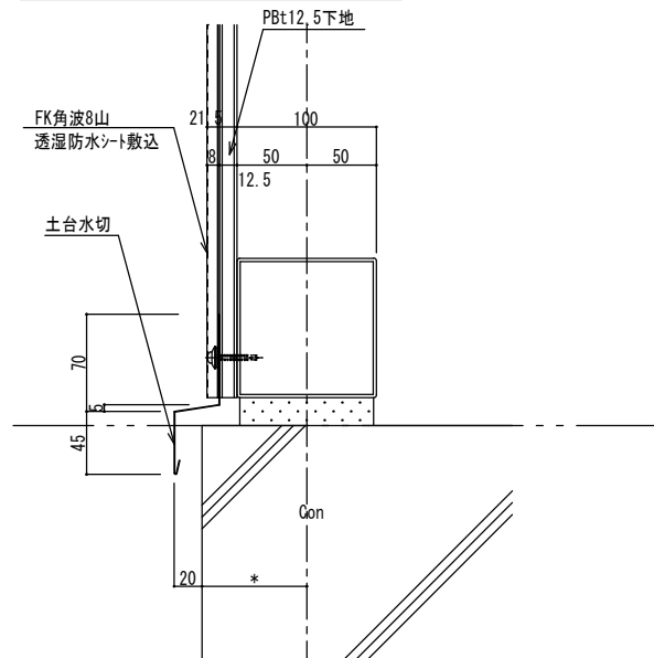
土台水切詳細図
