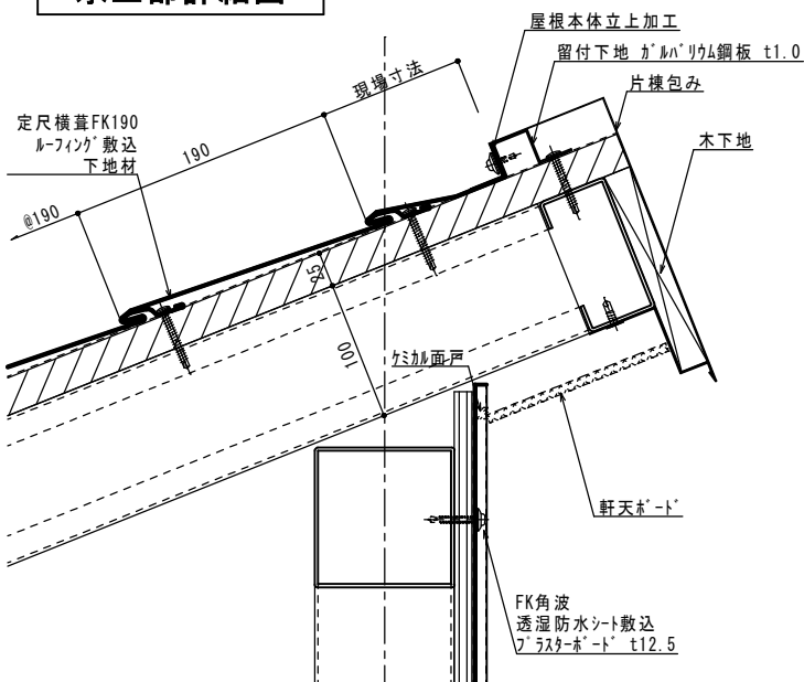
水上部詳細図
