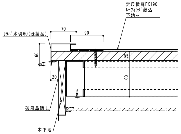
ケラハ'詳細図
