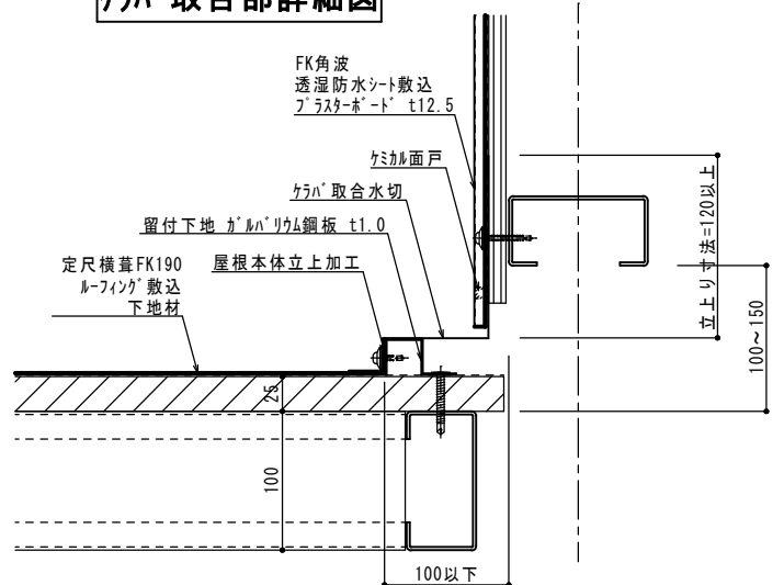
ケラハ'取合部詳細図
