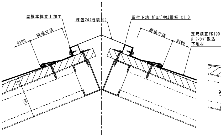
棟断面詳細図
