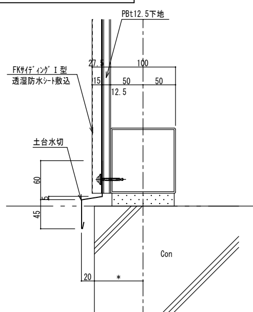
土台水切詳細図
