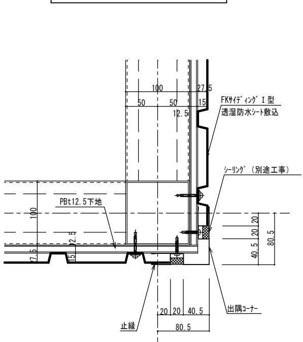
出隅コーナー詳細図
