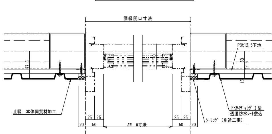
サッシ廻り (横断面) 詳細図
