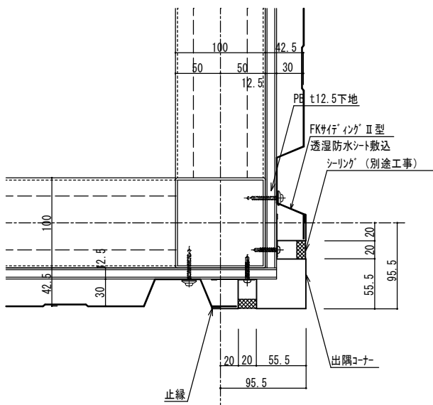
出隅コーナー詳細図
