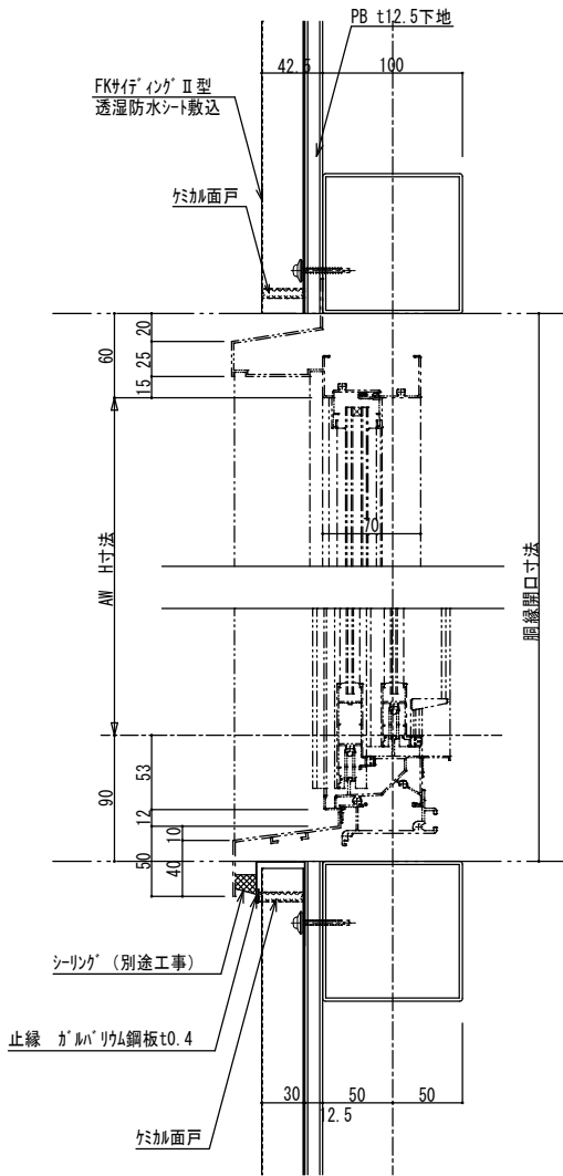
サッシ廻り(縦断面)詳細図
