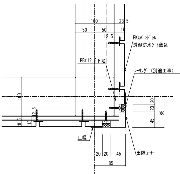
出隅コーナー詳細図
