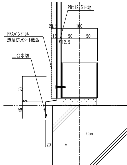
土台水切詳細図
