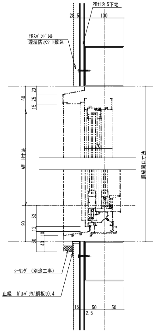
サッシ廻り(縦断面)詳細図
