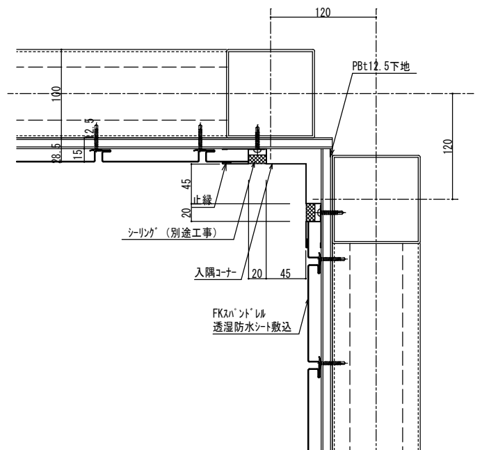
入隅コーナー詳細図
