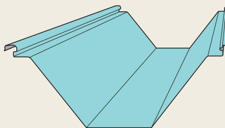
ヨドルーフ166ハゼ
