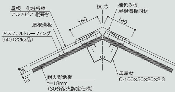
棟断面詳細図
