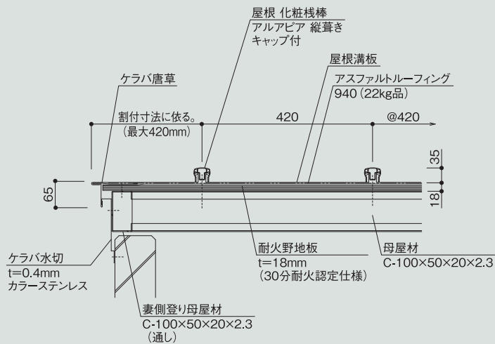
ケラバ詳細図
