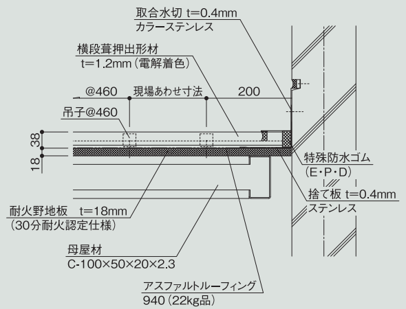
壁取合部詳細図
