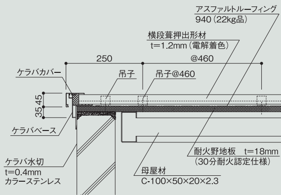
ケラバ詳細図
