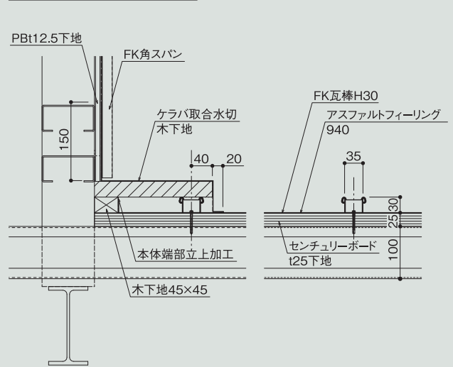
ケラバ取合部詳細図
