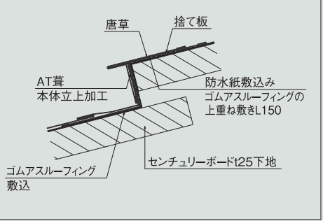
AT葺・瓦棒ジョイント部 拡大図
