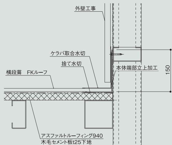
ケラバ取合部詳細図
