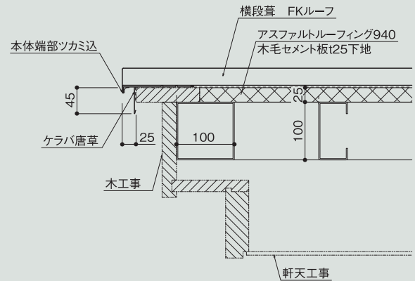
ケラバ詳細図
