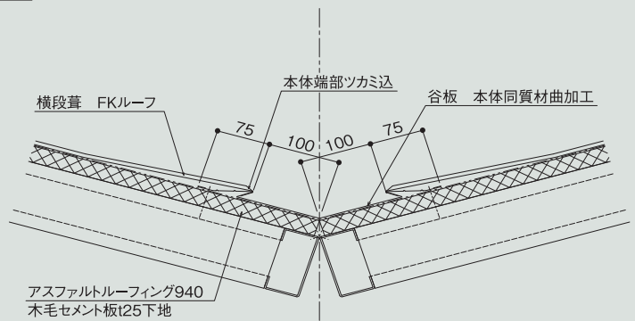
谷断面詳細図
