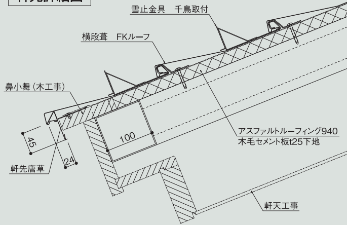
軒先詳細図
