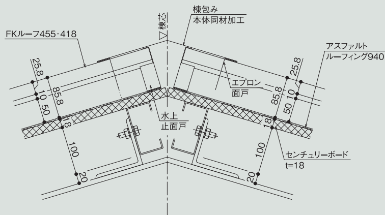
棟断面詳細図
