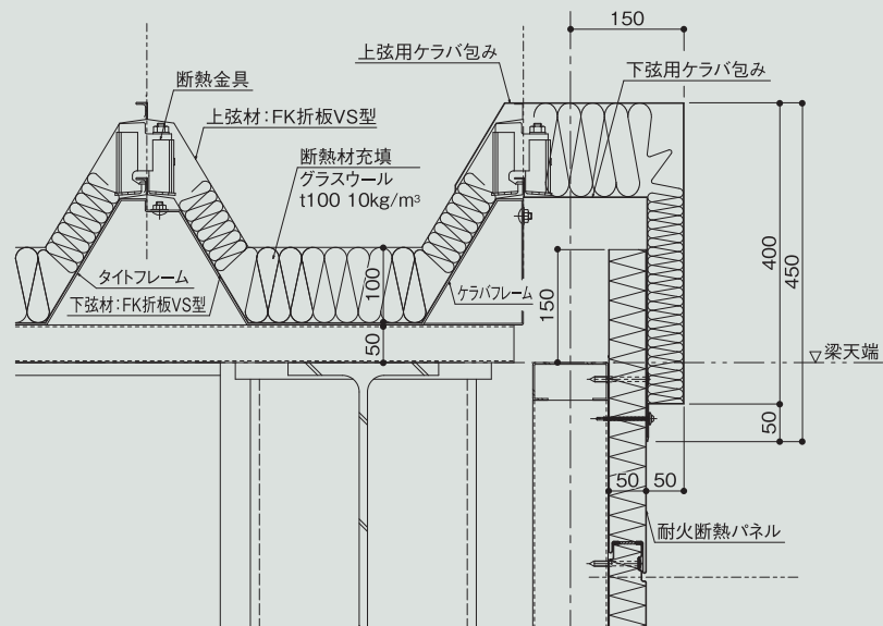
ケラバ取合部詳細図
