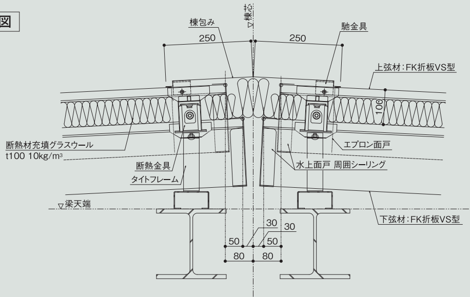
ケラバ包み詳細図
