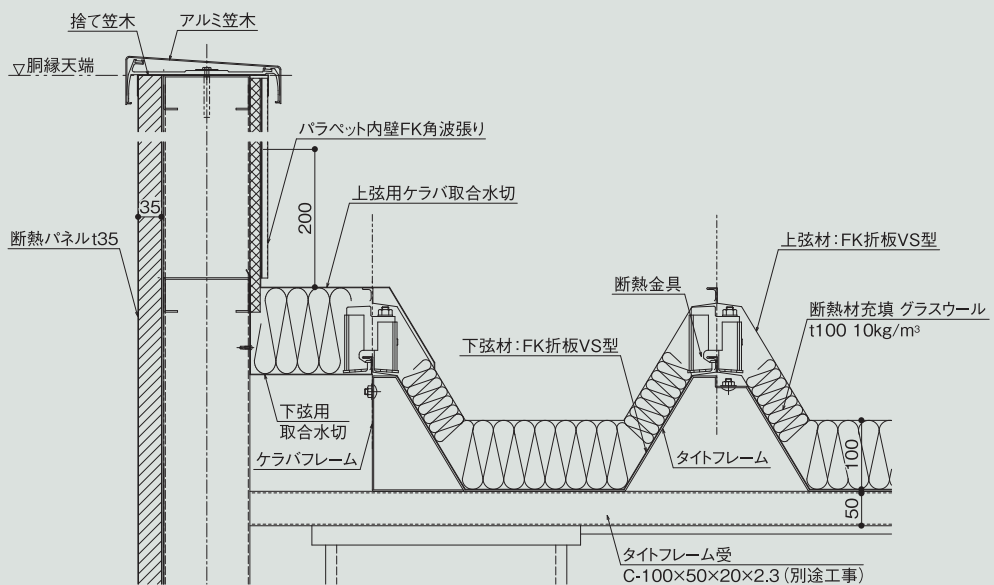
ケラバ取合部詳細図
