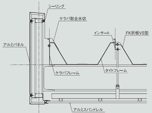
ケラバ取合部詳細図
