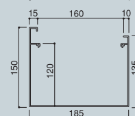
●軒15号 (受注生産)
